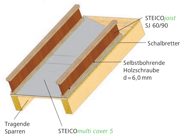
D12 Aufdachdämmung – Aufdoppelung mit STEICOjoist
