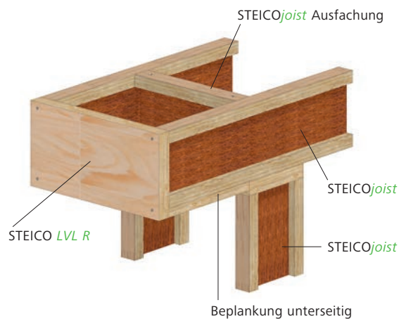
F6 Ausbildung von Kragarmen
