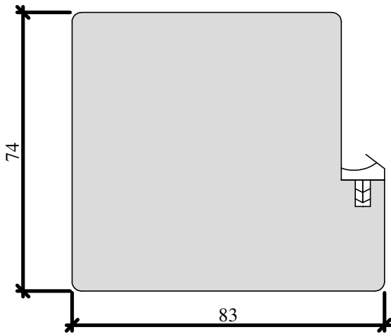
Blockrahmen stumpf einschlagend
