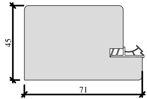
Blendrahmen auch RC2
